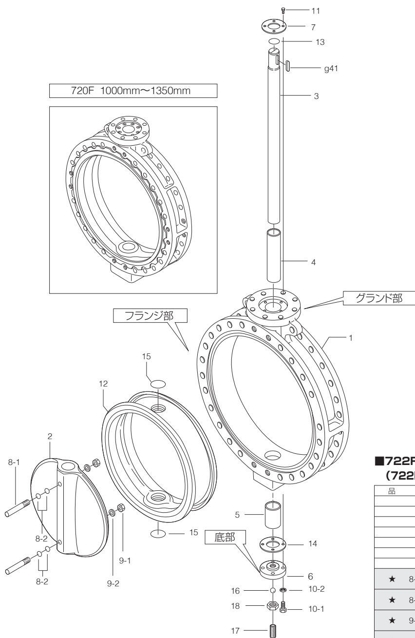
722F・720F 650mm~1350mm
