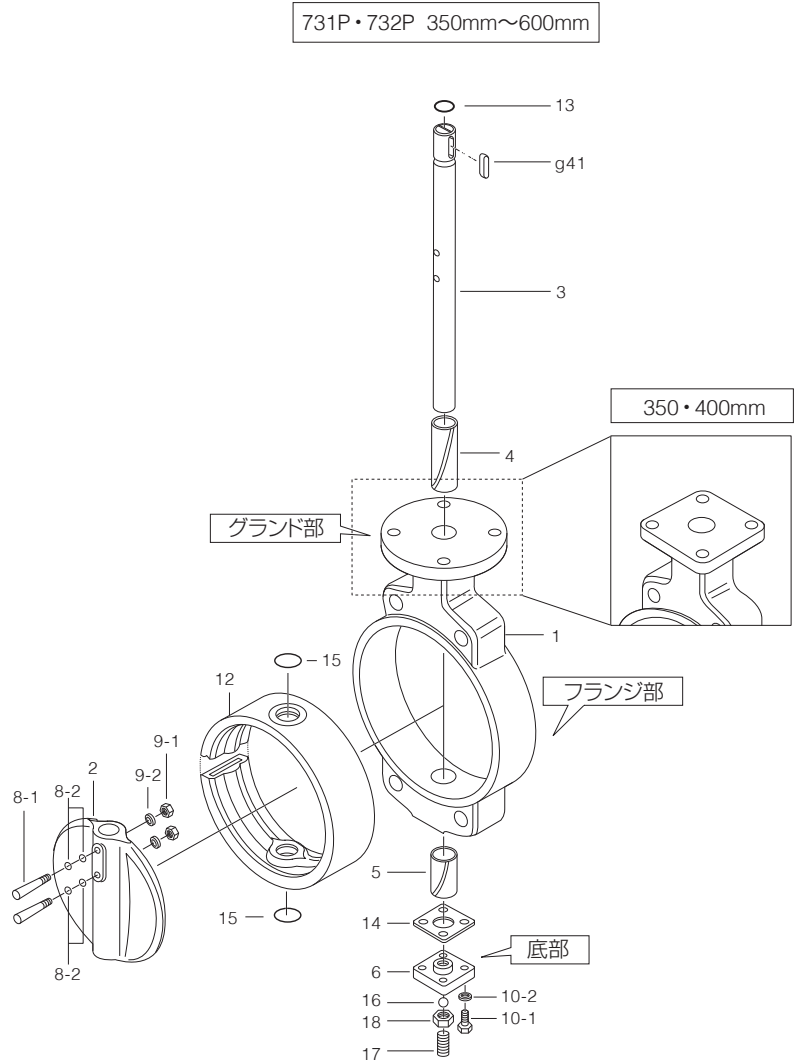
■731P・732P 本体部部品表 (350mm~600mm)
