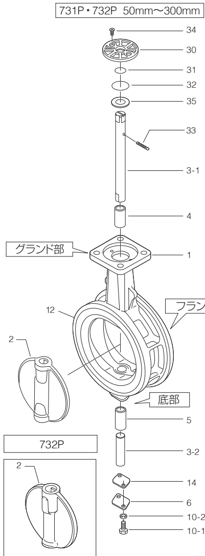
■731P・732P 本体部部品表 (50mm~300mm)
